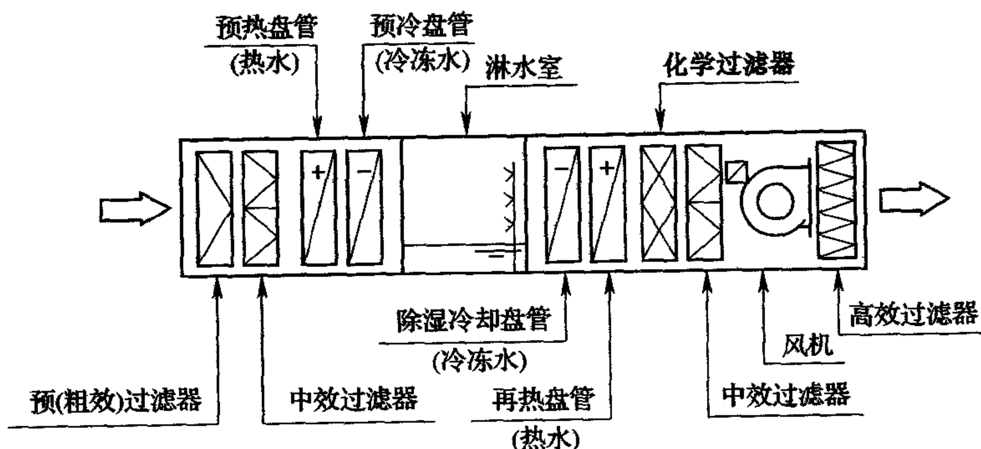
图 7 新风处理装置的示意
