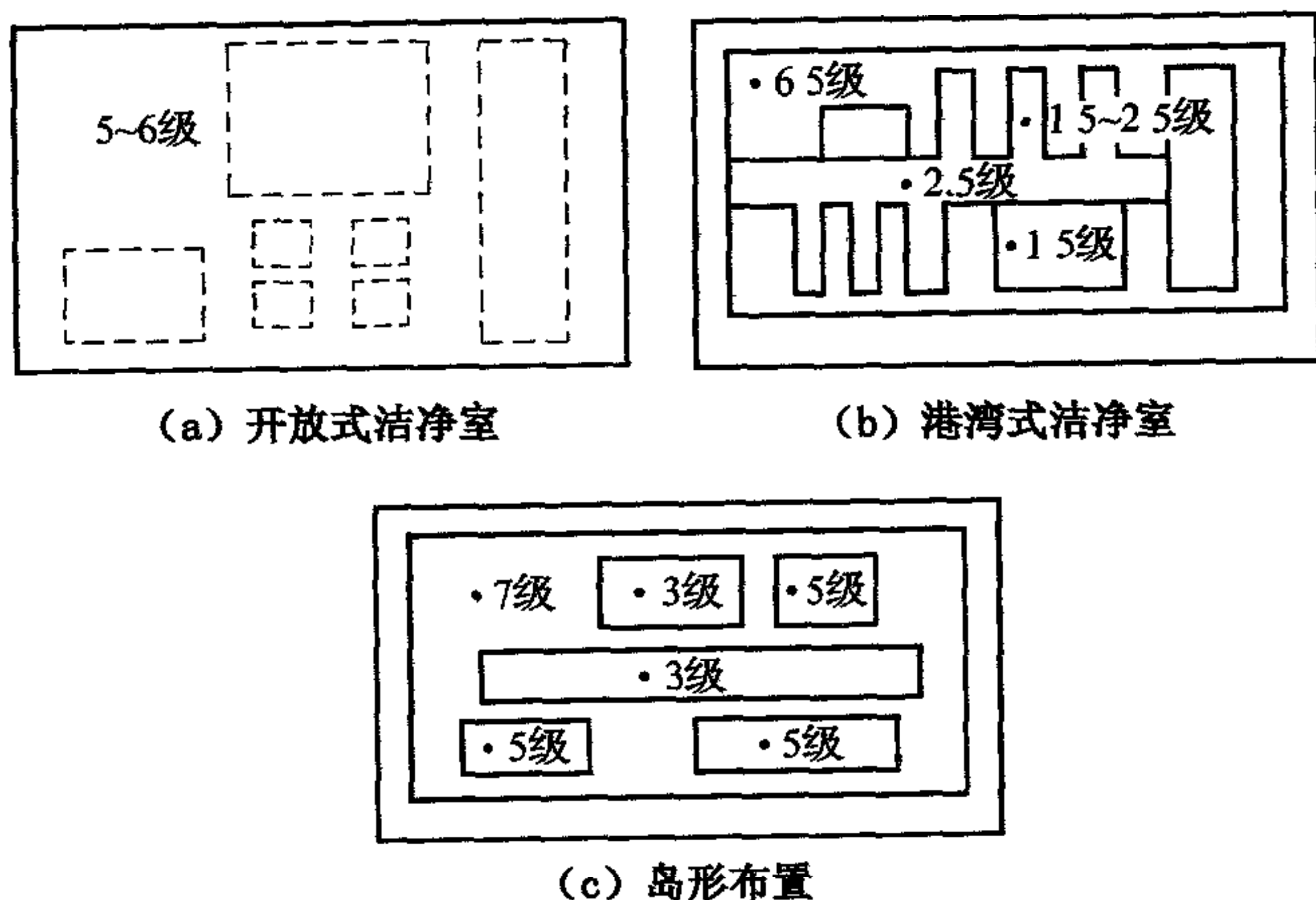
图 1 洁净室形式
