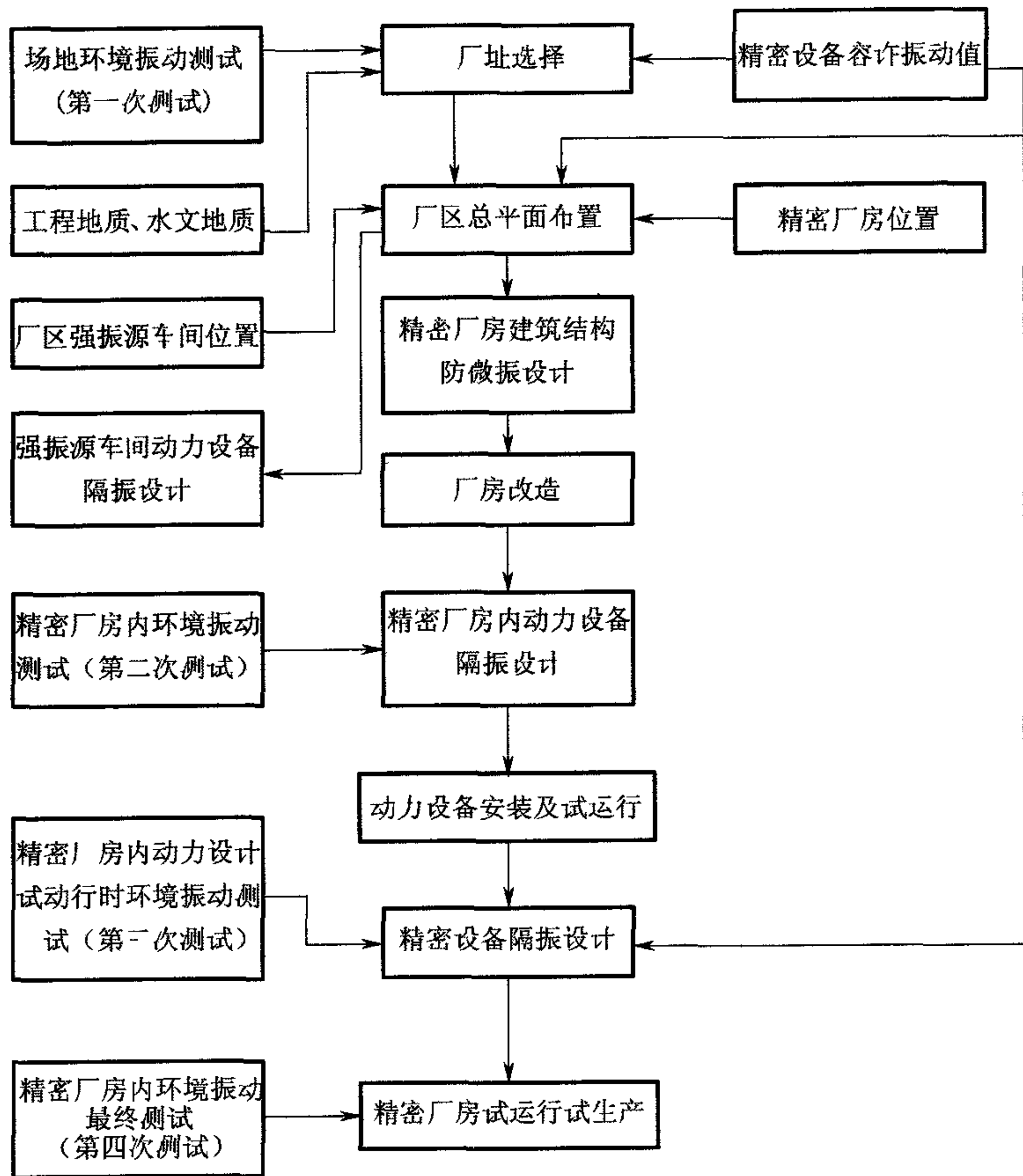
图 10 微振控制工程设计程序
